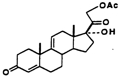
4,9(11)-Pregnadien-17a,21-diol-3,20-dione-21-acetate
